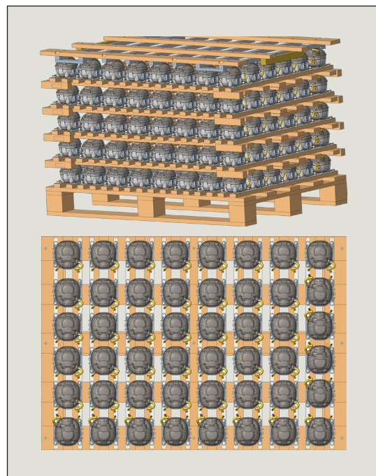
Fig. 2 New pallet, 240 compressors, 48 per layer
